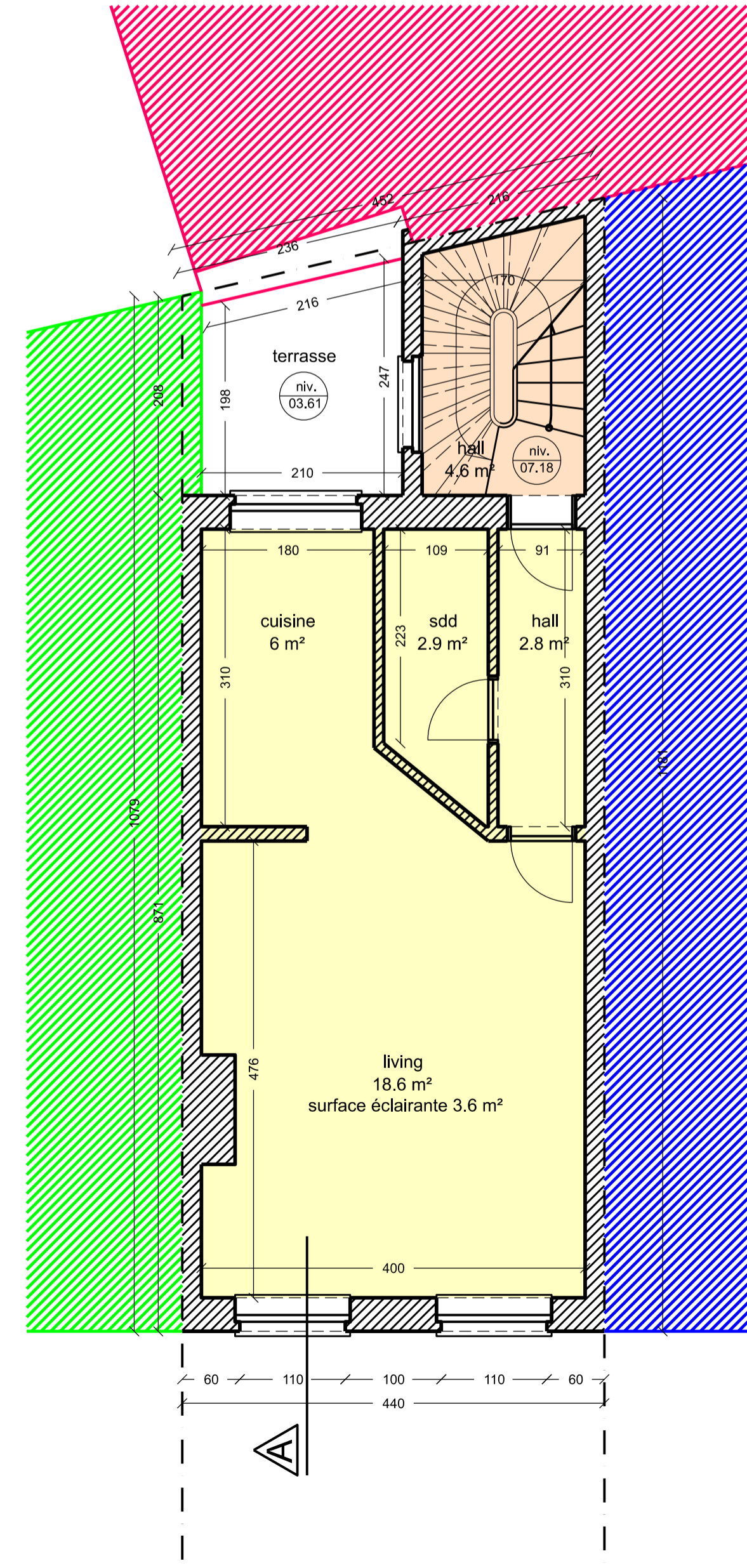
Plan 2ème
