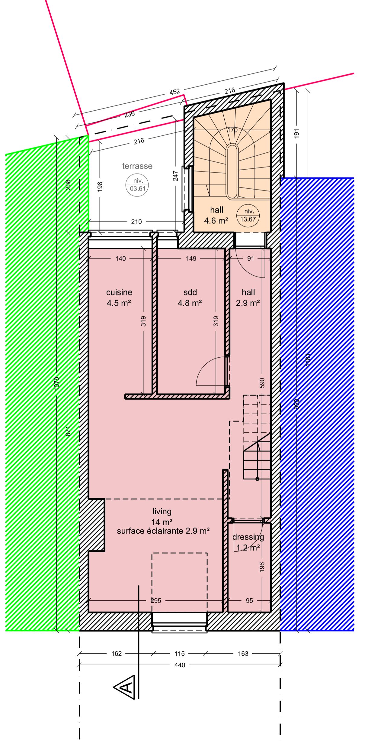
Plan 4ème
