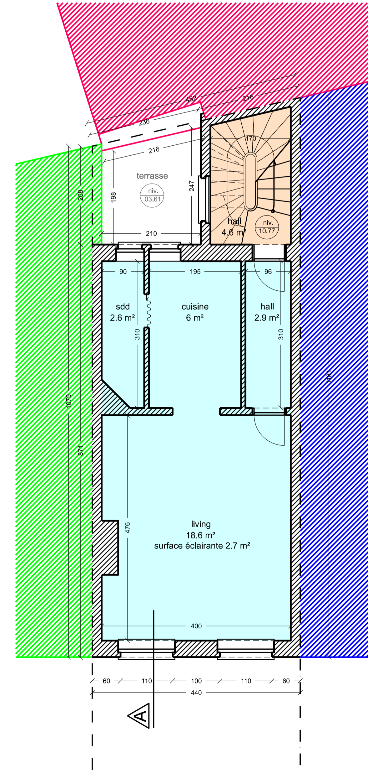
Plan 3ème
